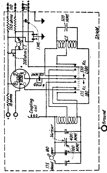
DayRad (Type 180)
